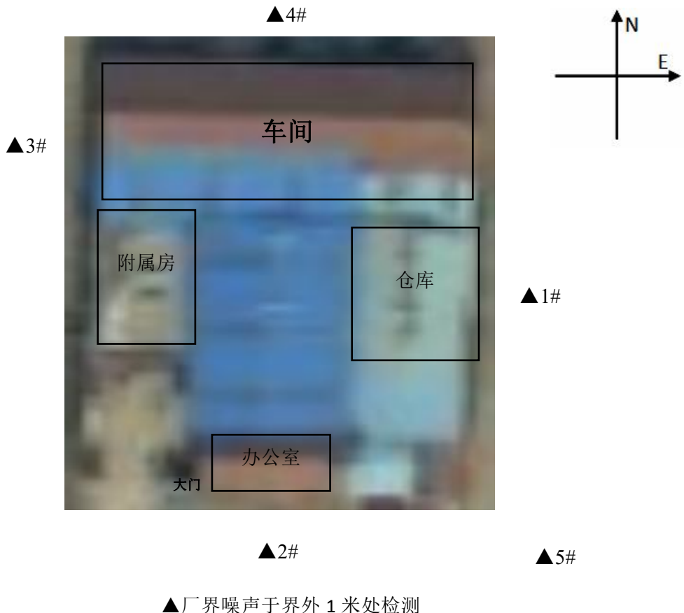
图6.4-1 噪声检测点位图
