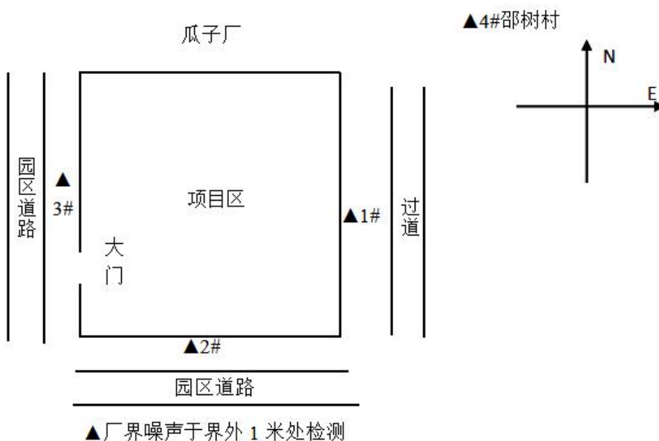
图 6.4-1 工业企业厂界环境噪声监测点布局
