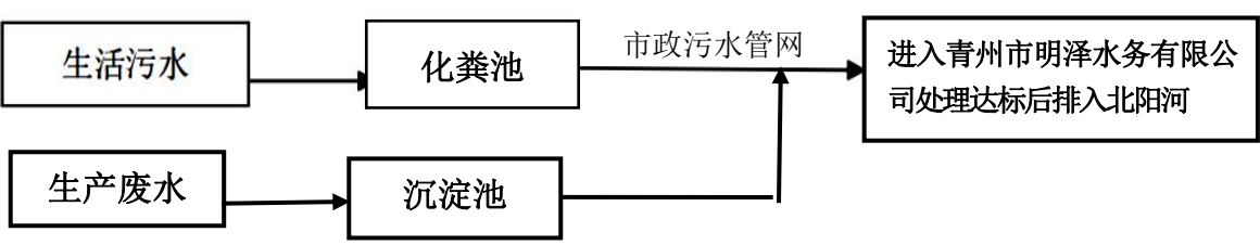
图 3.1-1 项目废水处理流程图
