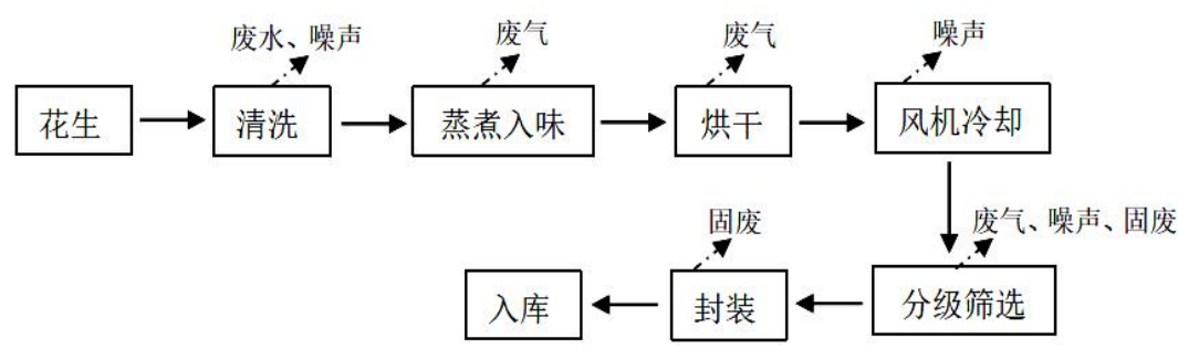
图 2.3-1 花生生产工艺及产污环节图
