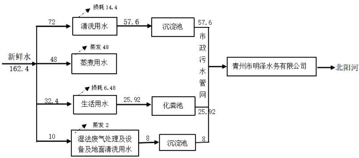
图 2.2-1 项目水平衡图 单位：m³/a
