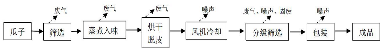
图 2.3-2 五香瓜子生产工艺及产污环节图
