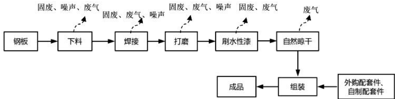
图 2.3-1 (1) 起重机工艺流程及产污环节示意图
