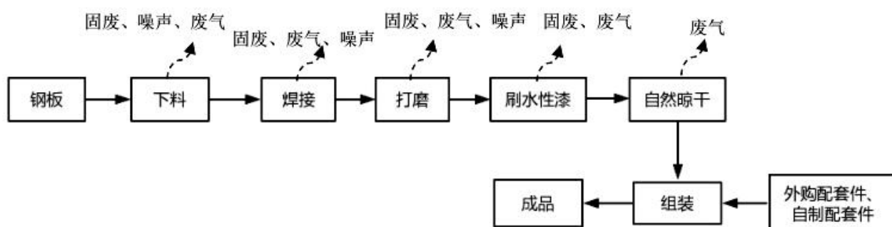
图一 起重机工艺流程及产污环节示意图
