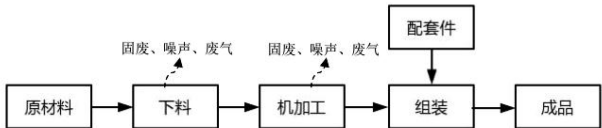
图 2.3-1 (2) 备件工艺流程及产污环节示意图
