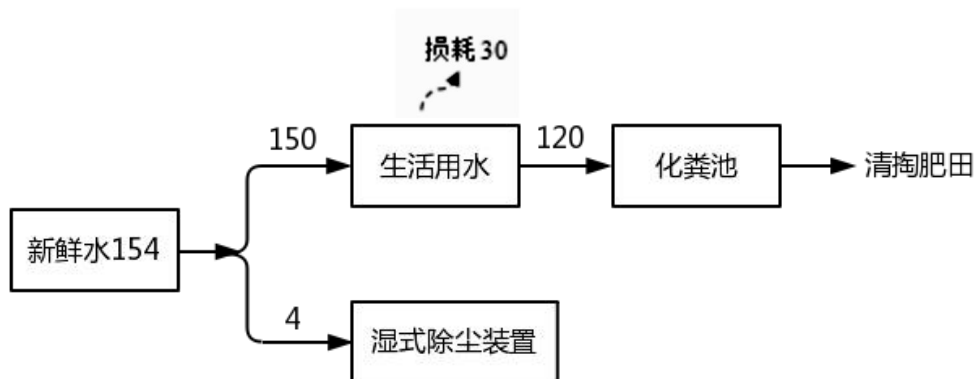
图 2.2-2 项目水量平衡图
