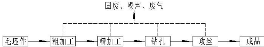
图 2.3-1 农用机械配件工艺流程及产污环节示意图
