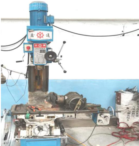
铣床
