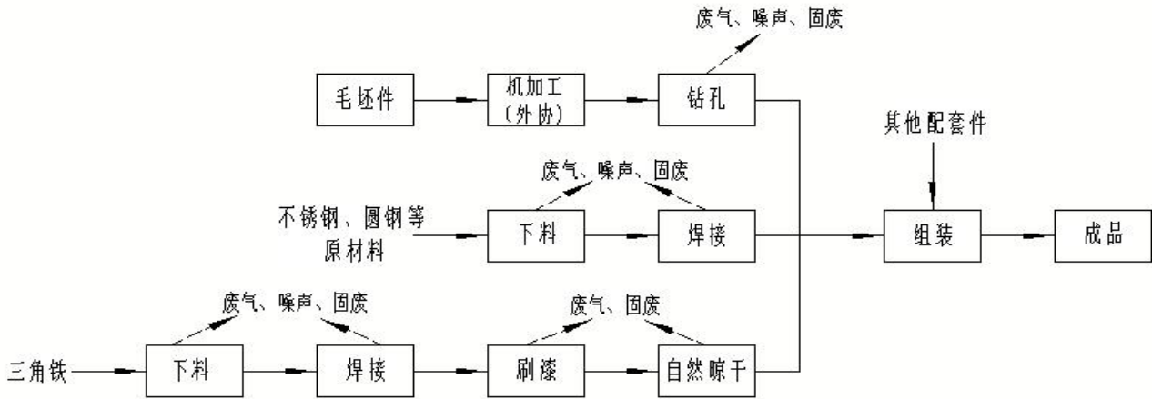
图 2.3-1 工艺流程及产污环节示意图
