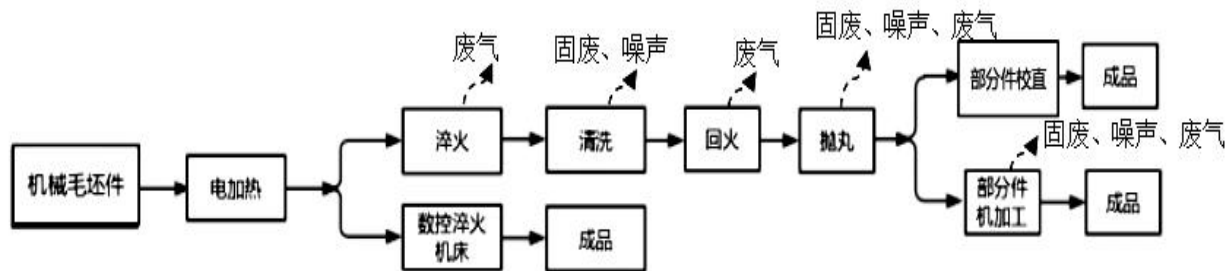
图 2.3-1 生产工艺流程及产污环节示意图
