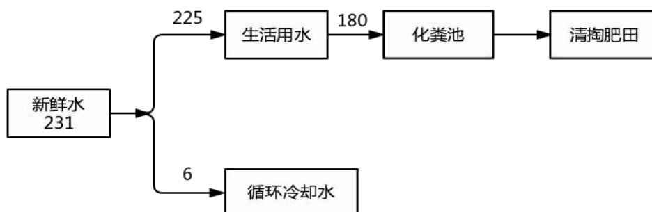
图 2.2-2 项目水量平衡图
