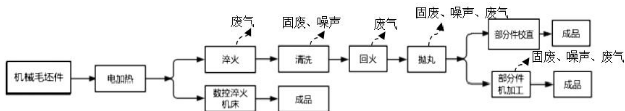
生产流程图及产污环节示意图
