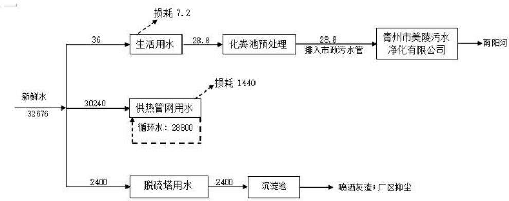
图 2.2-1 项目水平衡图 单位：m³/a
