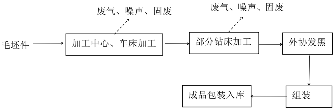
图2.3-1 控制阀生产工艺流程及产污环节示意图
