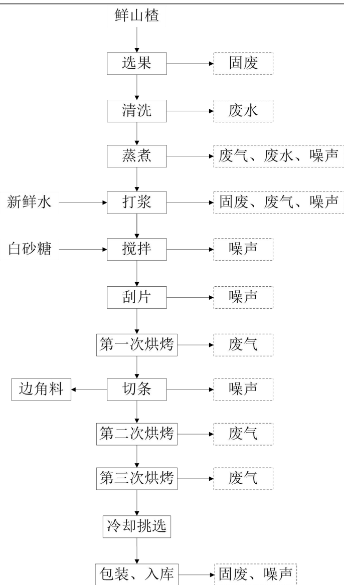
图 2 山楂条生产工艺流程及产污环节图
