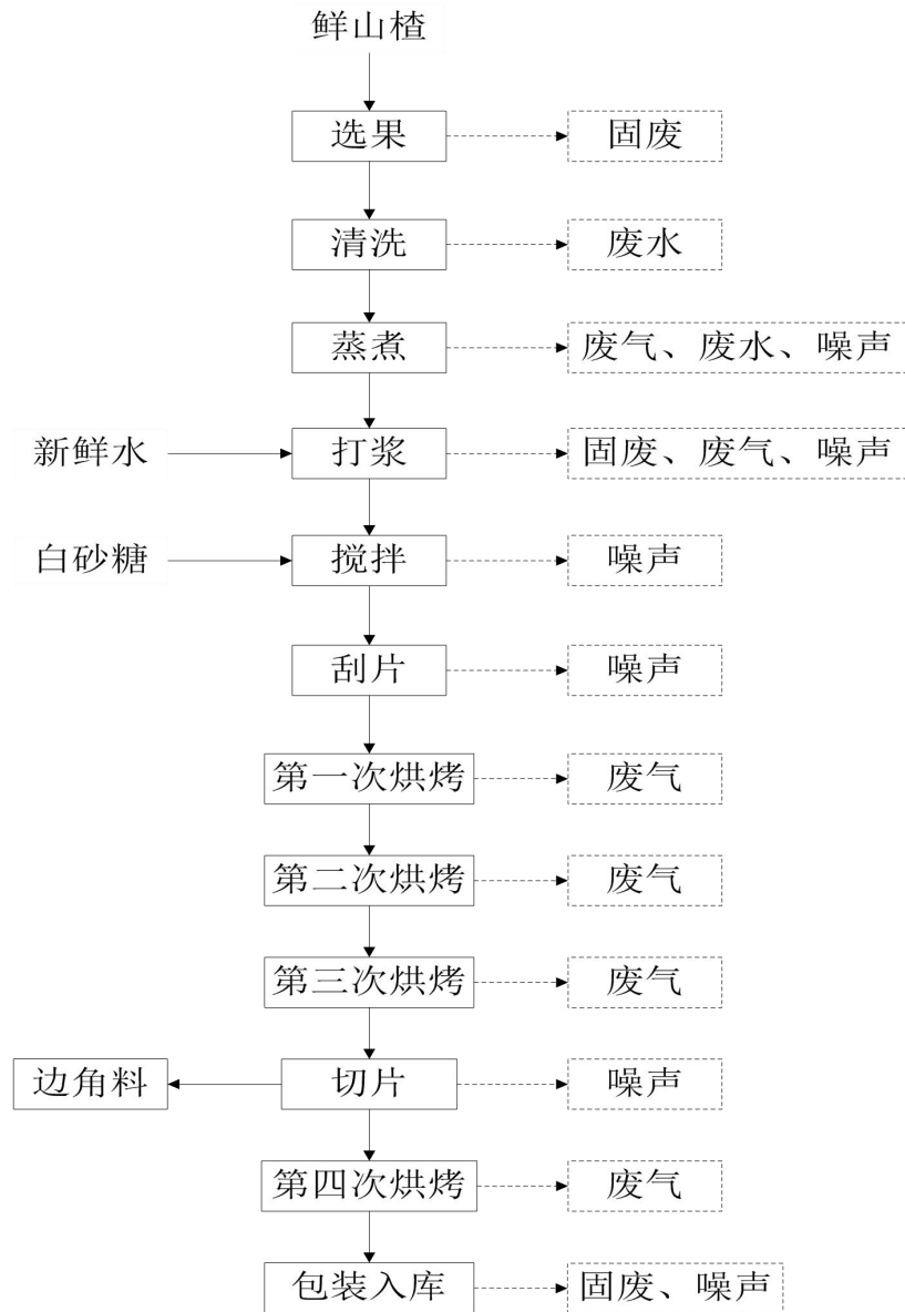
图 2.3-1 山楂片生产工艺流程及产污环节图
