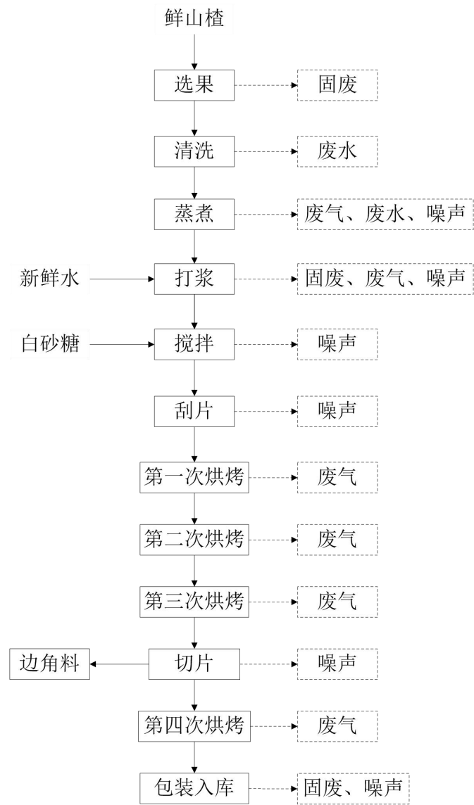
图 1 山楂片生产工艺流程及产污环节图
