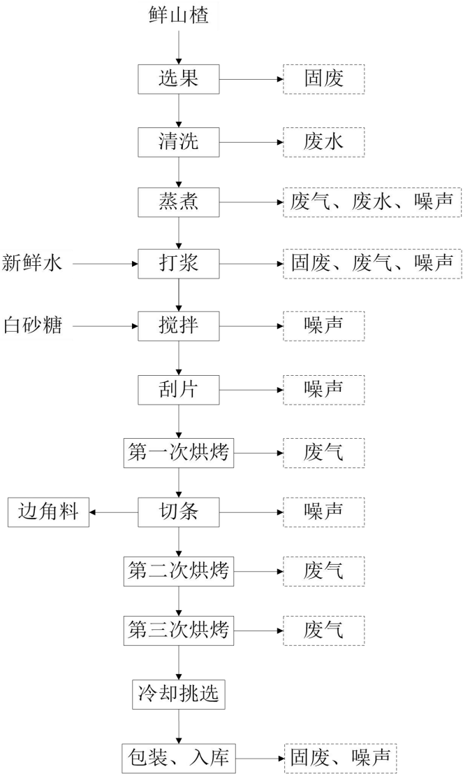
图 2.3-2 山楂条生产工艺流程及产污环节图
