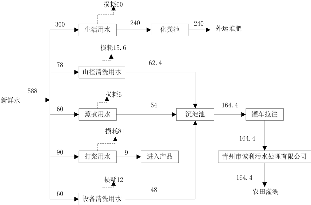
本项目水量平衡图：
