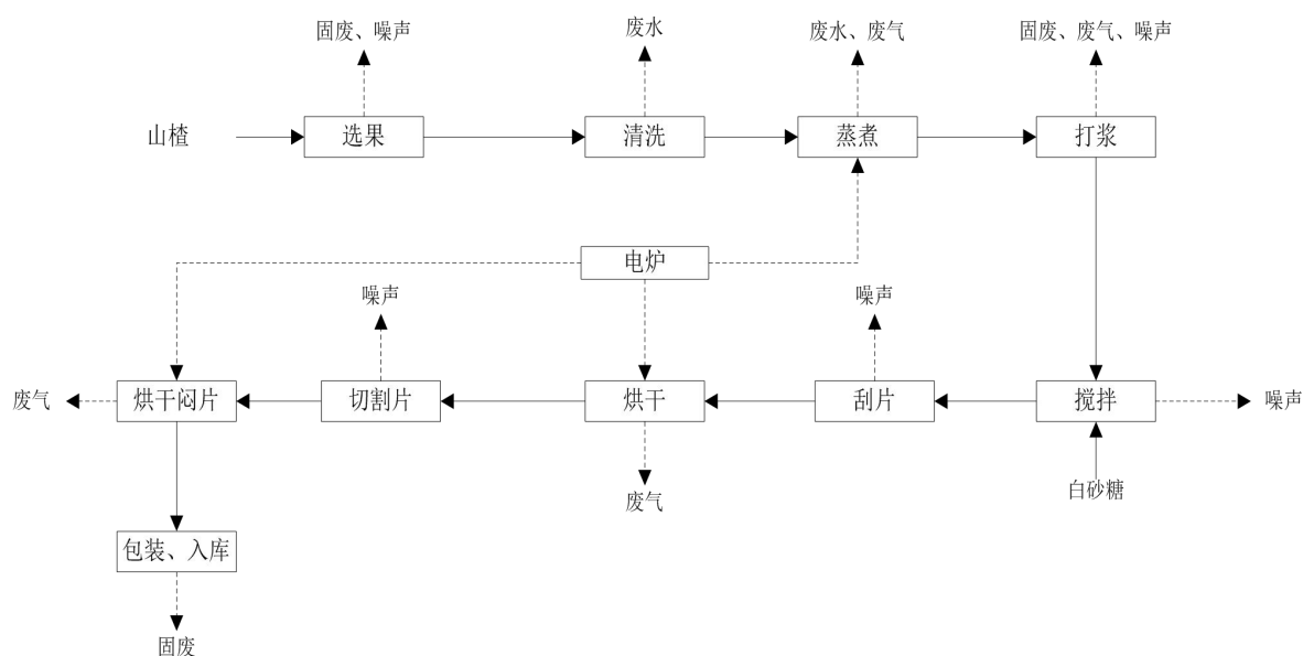
图 1 工艺流程及产污环节示意图
