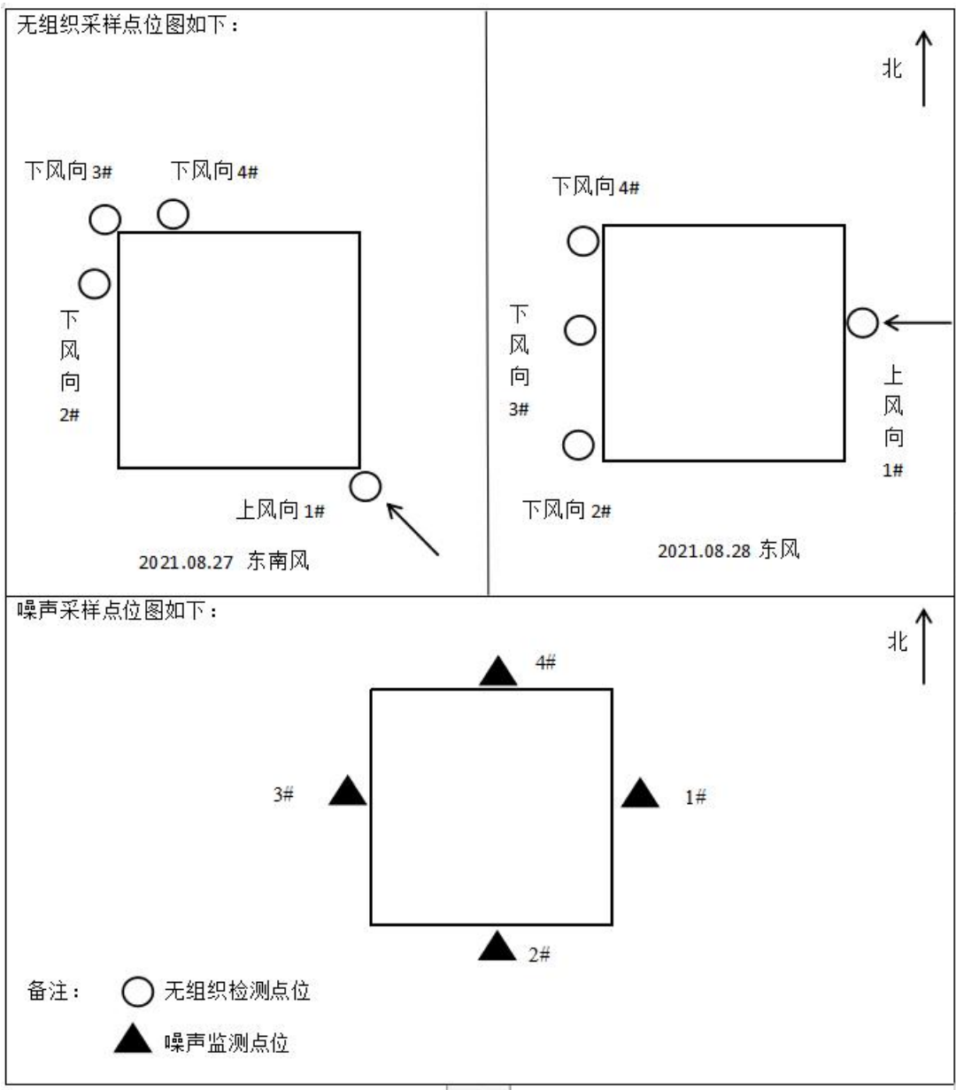
图 6-1 废气和噪声检测点位图
