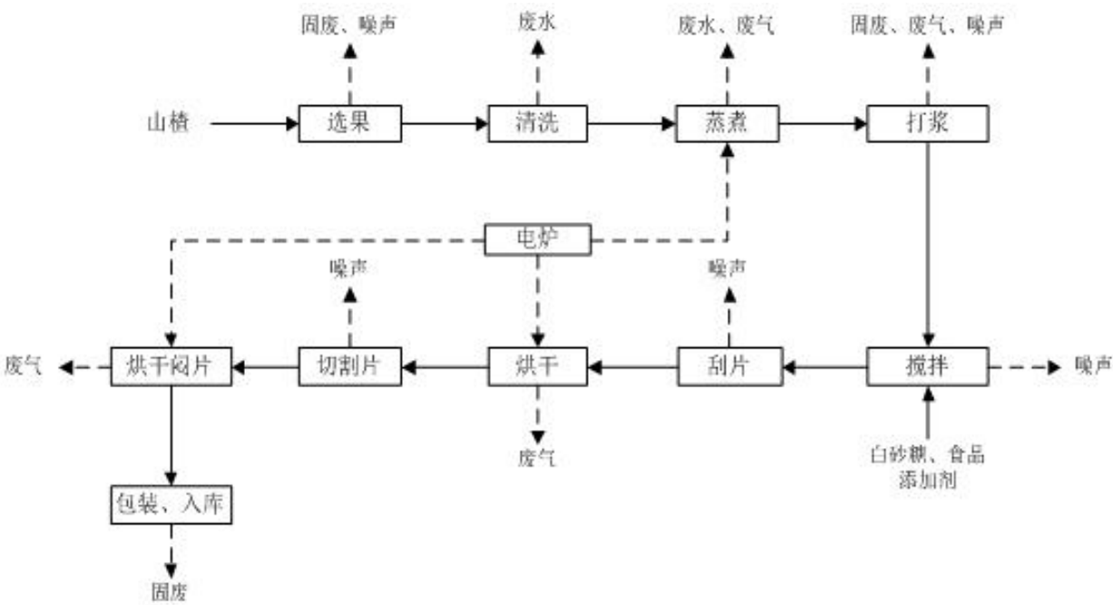
图 1 山植片生产工艺流程及产污环节图
