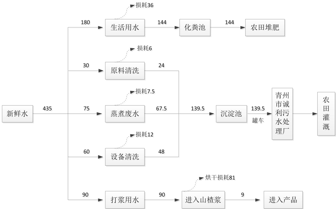
图 2.2-2 项目水量平衡图 单位：m 3 /a
