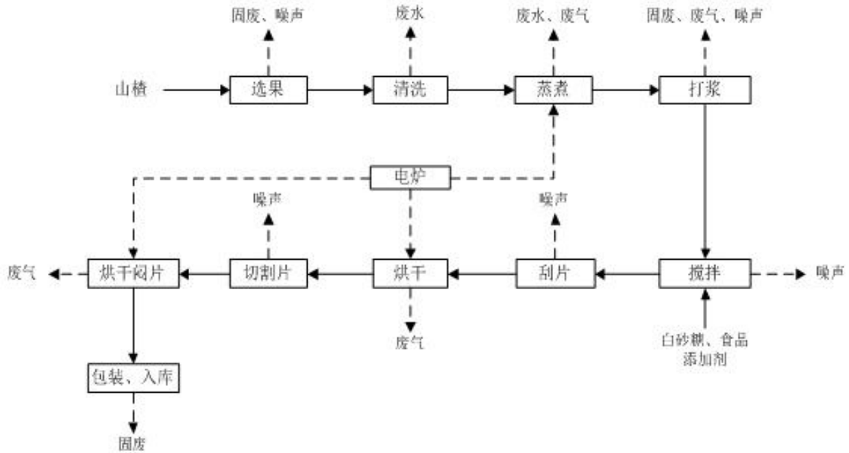
图 2.3-1 山楂片生产工艺流程及产污环节图
