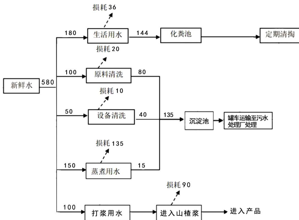
图 2.2-2 项目水量平衡图 单位：m 3 /a
