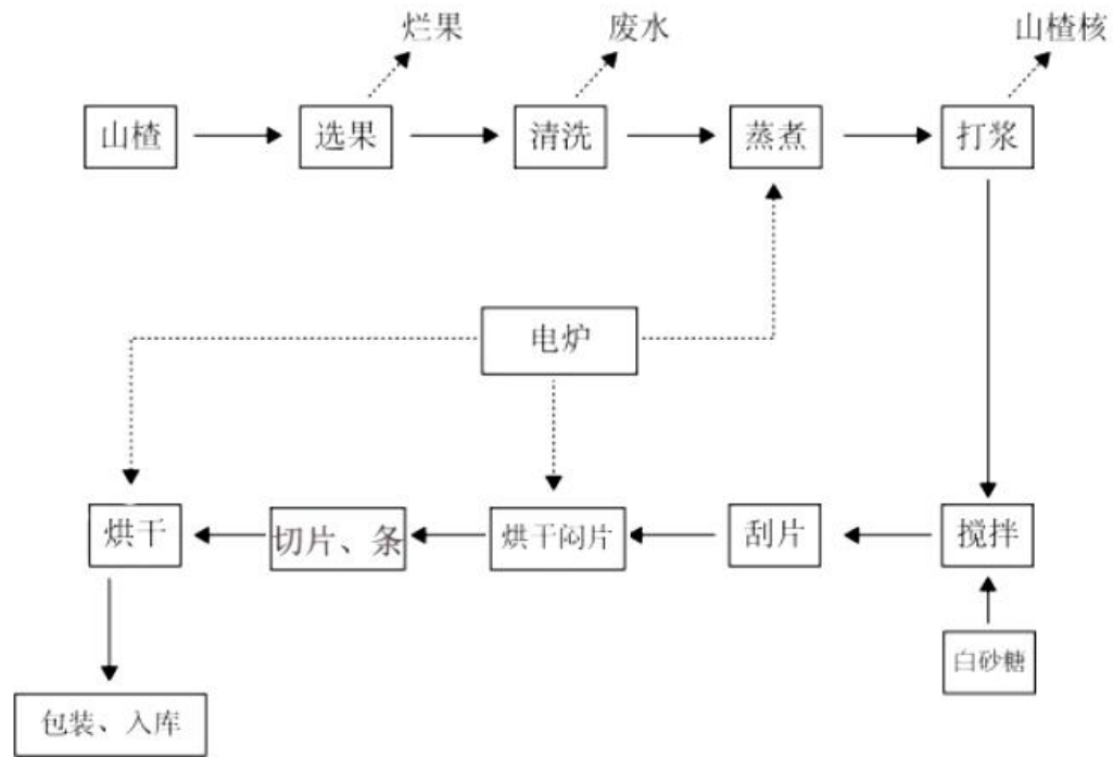
图 2.3-1 工艺流程及产污环节示意图
