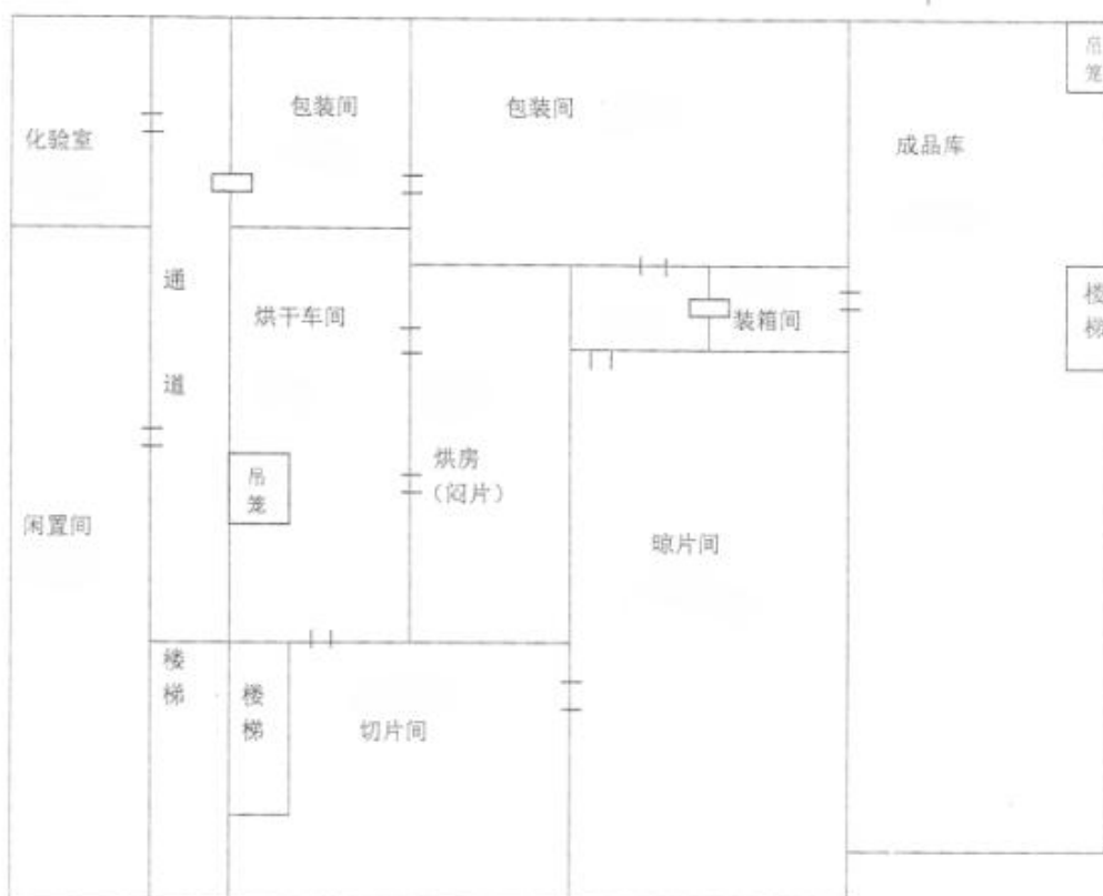
图 2 项目平面布置图 比例尺 1:500
