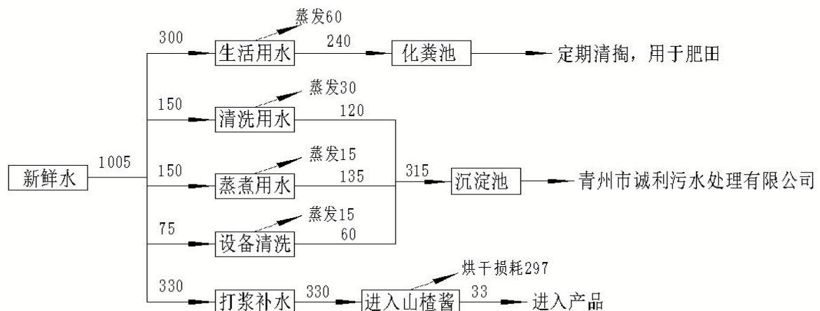
图 2.2-2 项目水量平衡图
