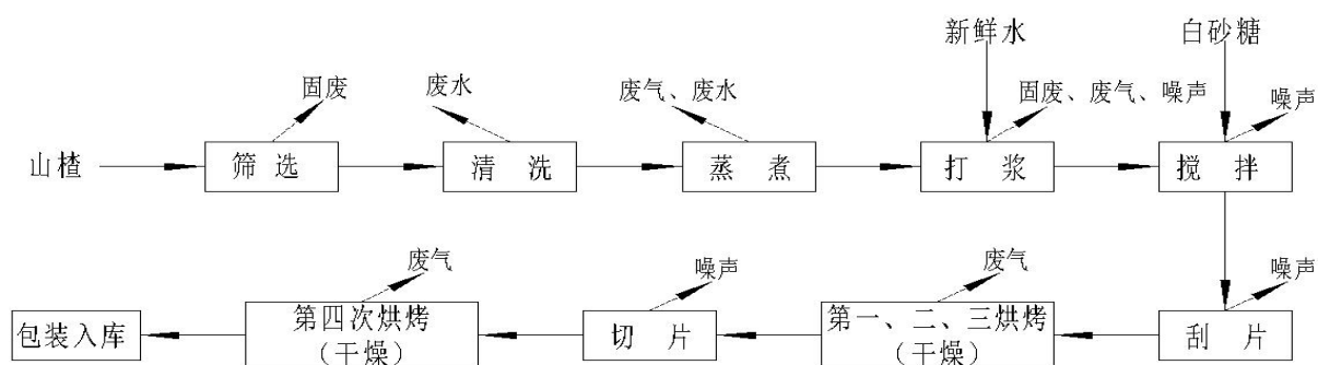
图 1 工艺流程及产污环节示意图
