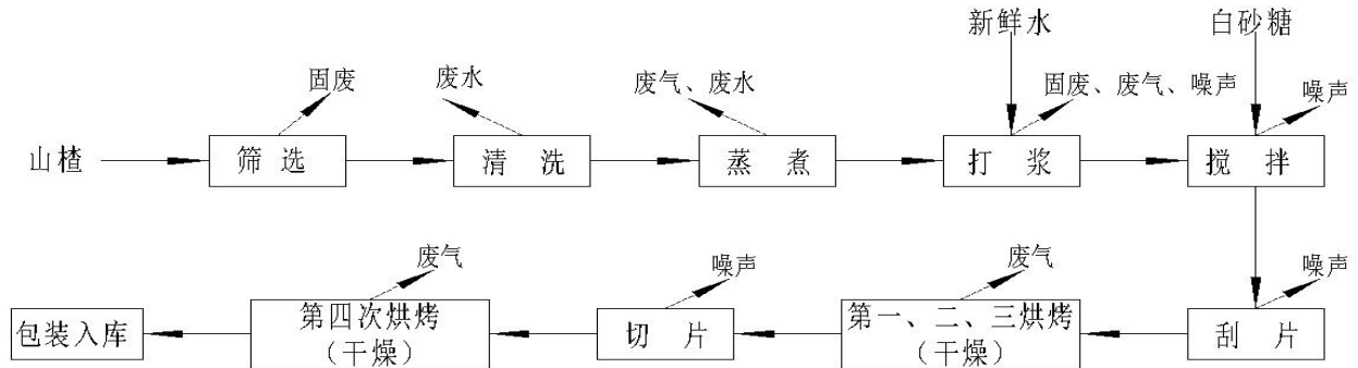
图 2.3-1 工艺流程及产污环节示意图
