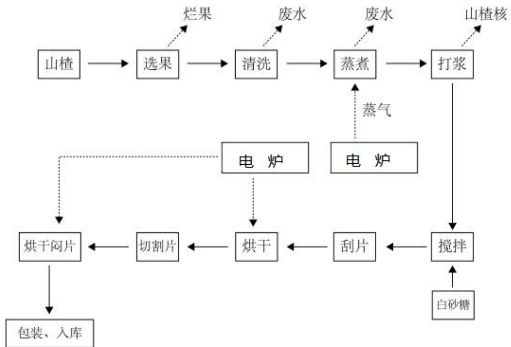
图 2.3-1 山楂片生产工艺流程及产污环节图
