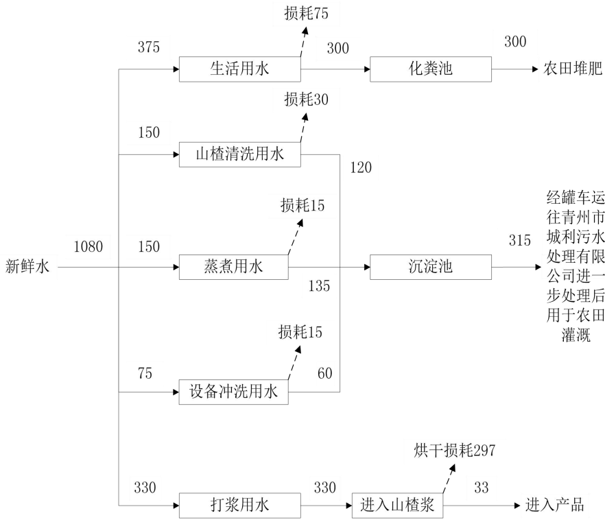
图 2.2-2 项目水量平衡图 单位：m³/a
