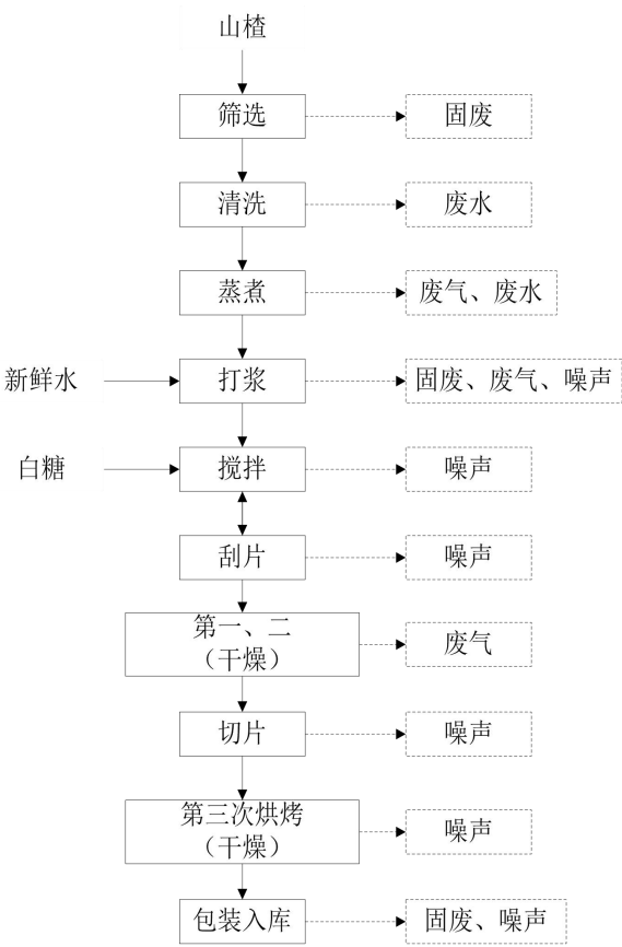
图 1 工艺流程及产污环节示意图
