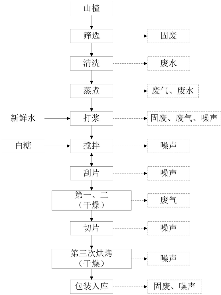
图 2.3-1 工艺流程及产污环节示意图
