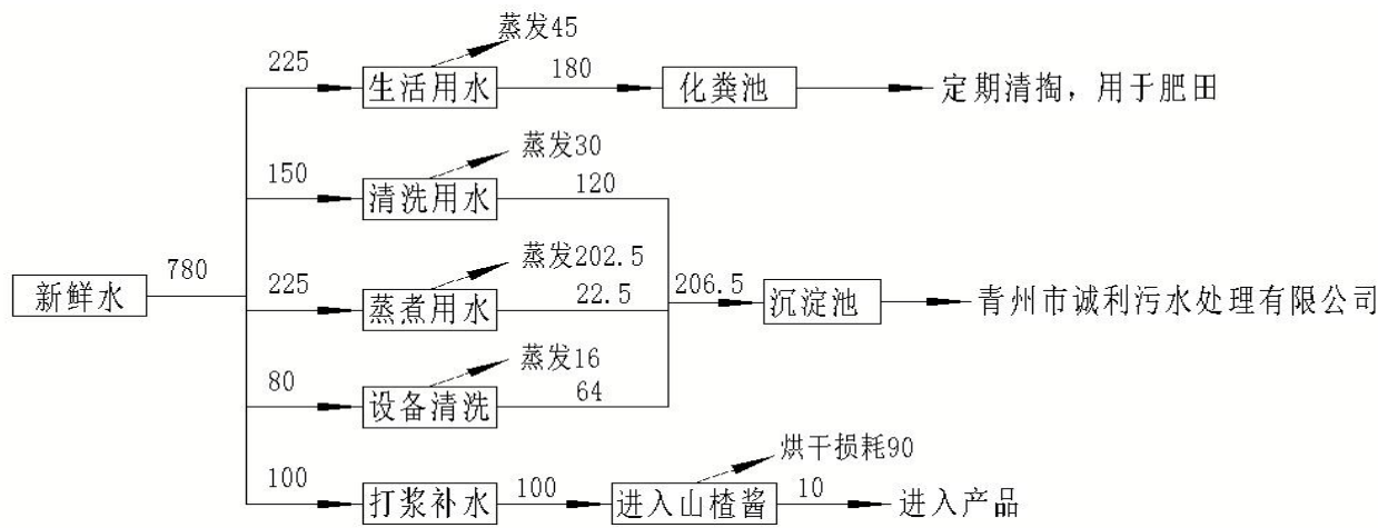
图 2.2-2 项目水量平衡图 单位：m 3 /a
