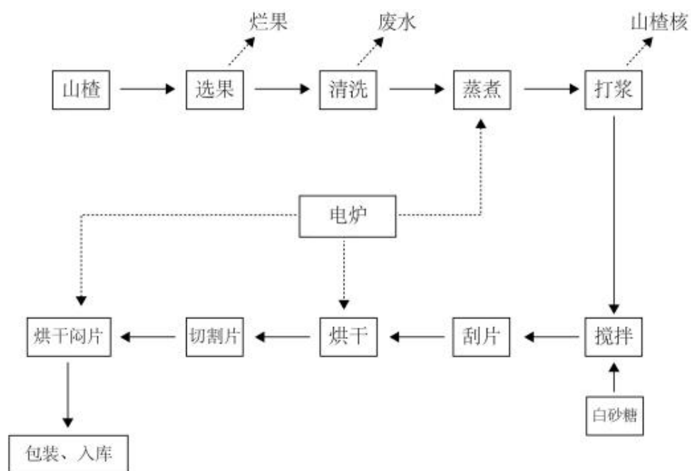
图 1 工艺流程及产污环节示意图
