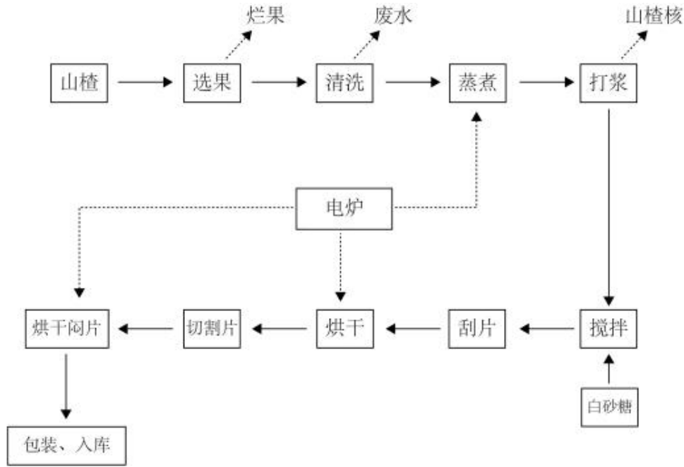
图 2.3-1 工艺流程及产污环节示意图
