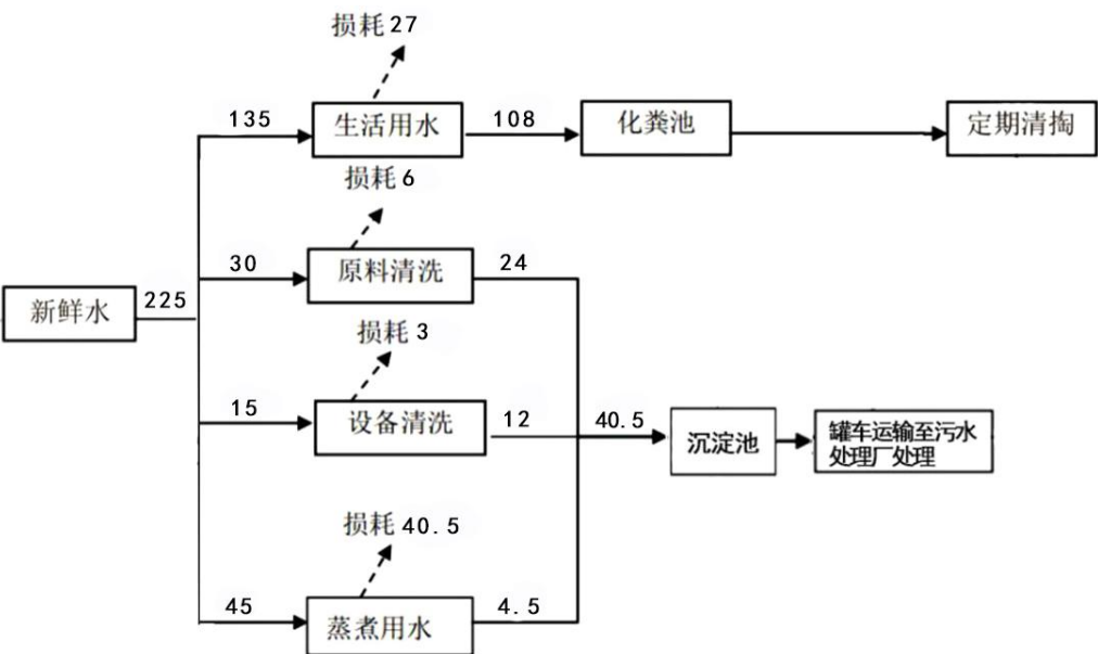
图 2.2-2 项目水量平衡图 单位：m³/a
