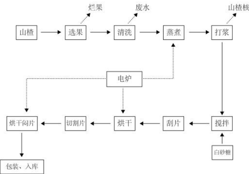
图 2.3-1 工艺流程及产污环节示意图
