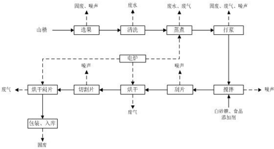
图 1 工艺流程及产污环节示意图
