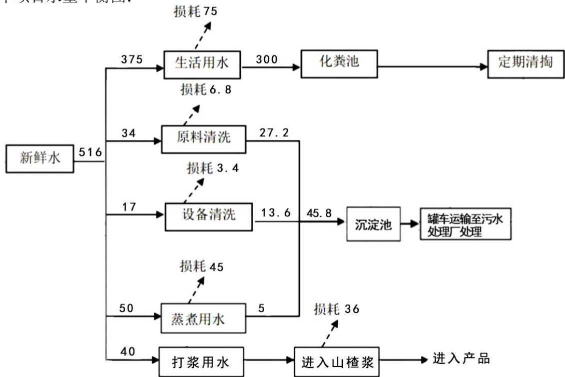
图 2.2-2 项目水量平衡图 单位：m³/a
