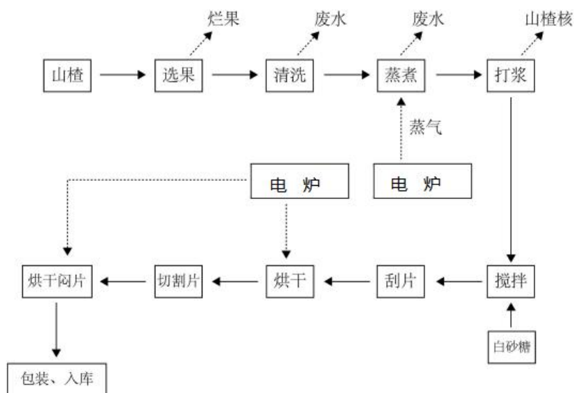
图 1 工艺流程及产污环节示意图
