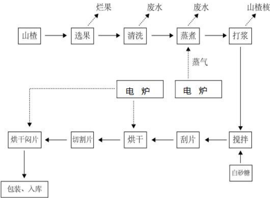
图 2.3-1 工艺流程及产污环节示意图
