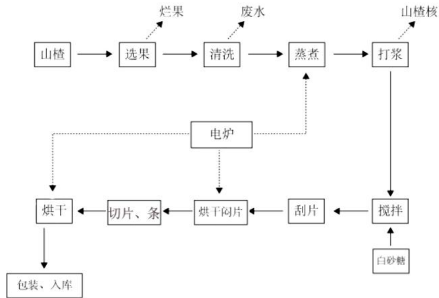
图 1 工艺流程及产污环节示意图
