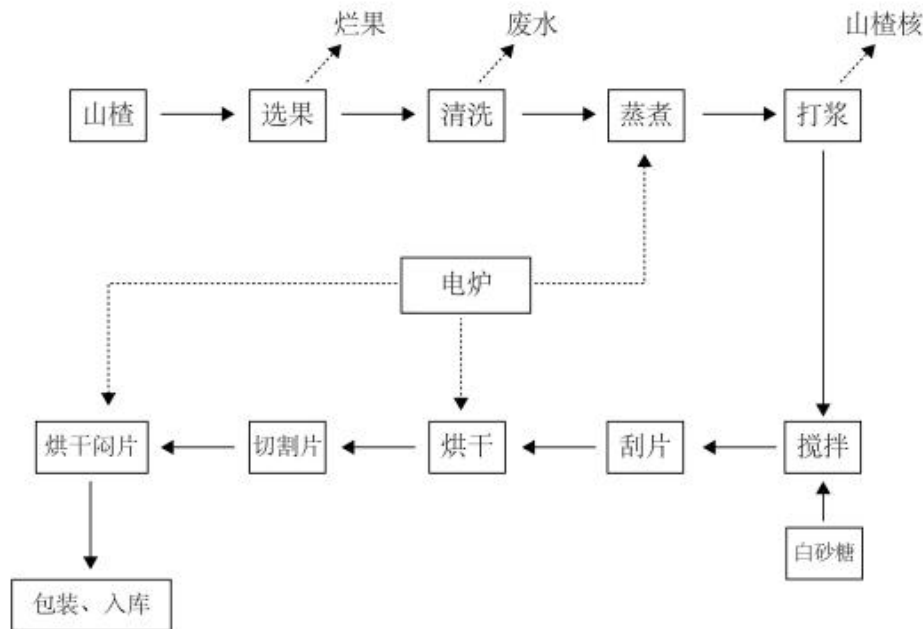
图 2.3-1 工艺流程及产污环节示意图
