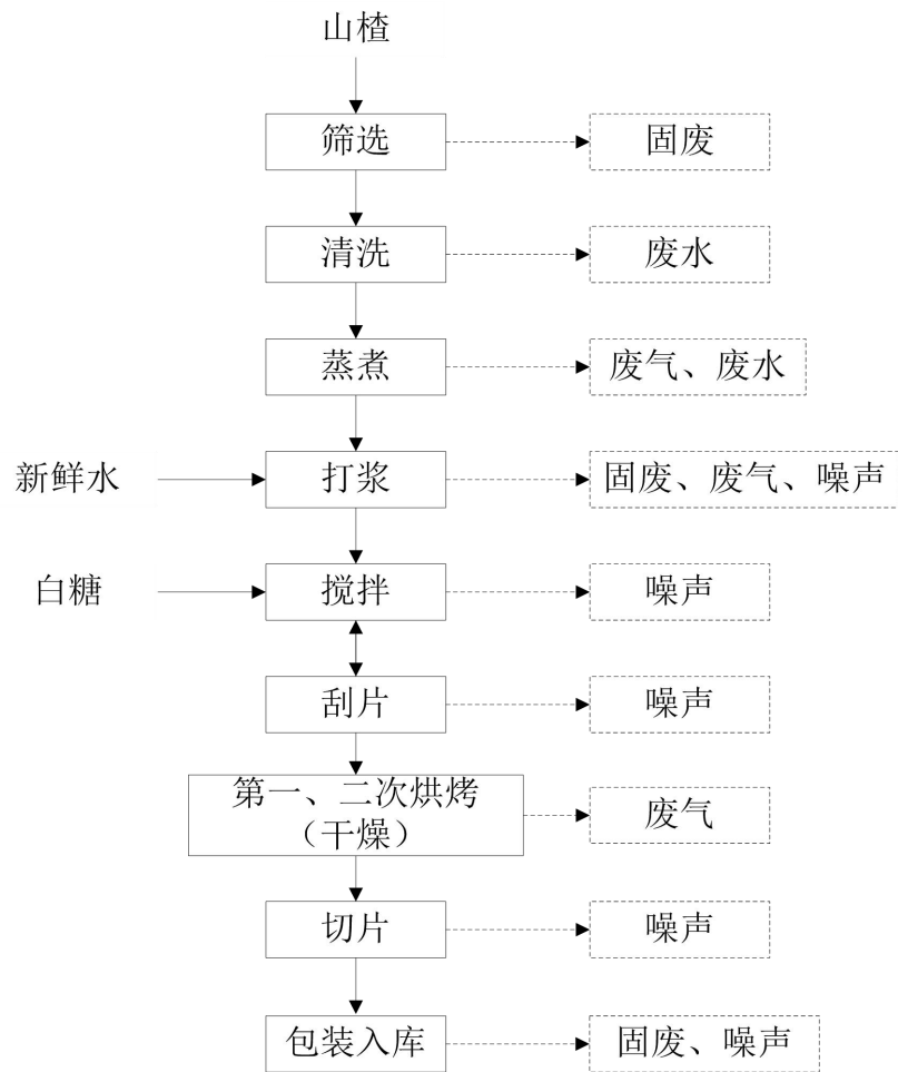
图 2.3-1 工艺流程及产污环节示意图
