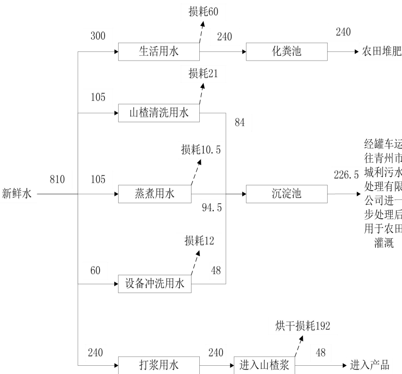
图 2.2-2 项目水量平衡图 单位：m 3 /a
