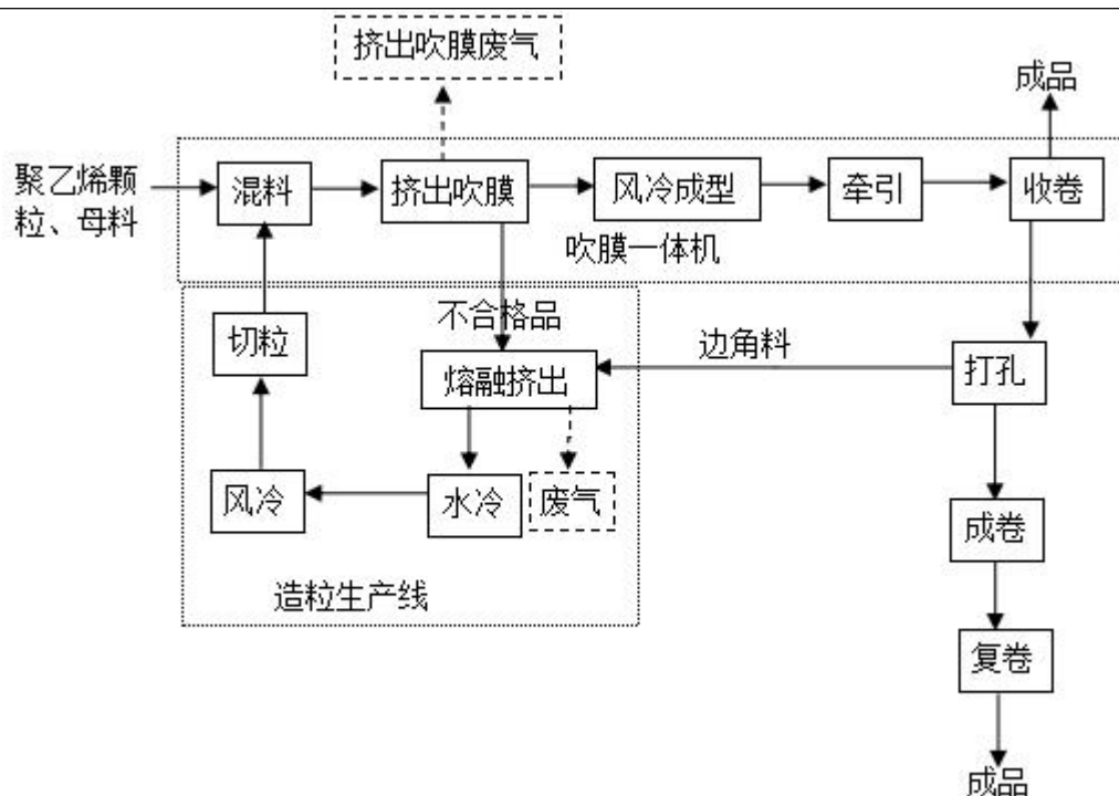
图 2-2 项目塑料薄膜生产工艺及产污环节图
