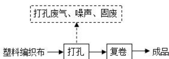
图 2-3 项目塑料编织布生产工艺及产污环节图
