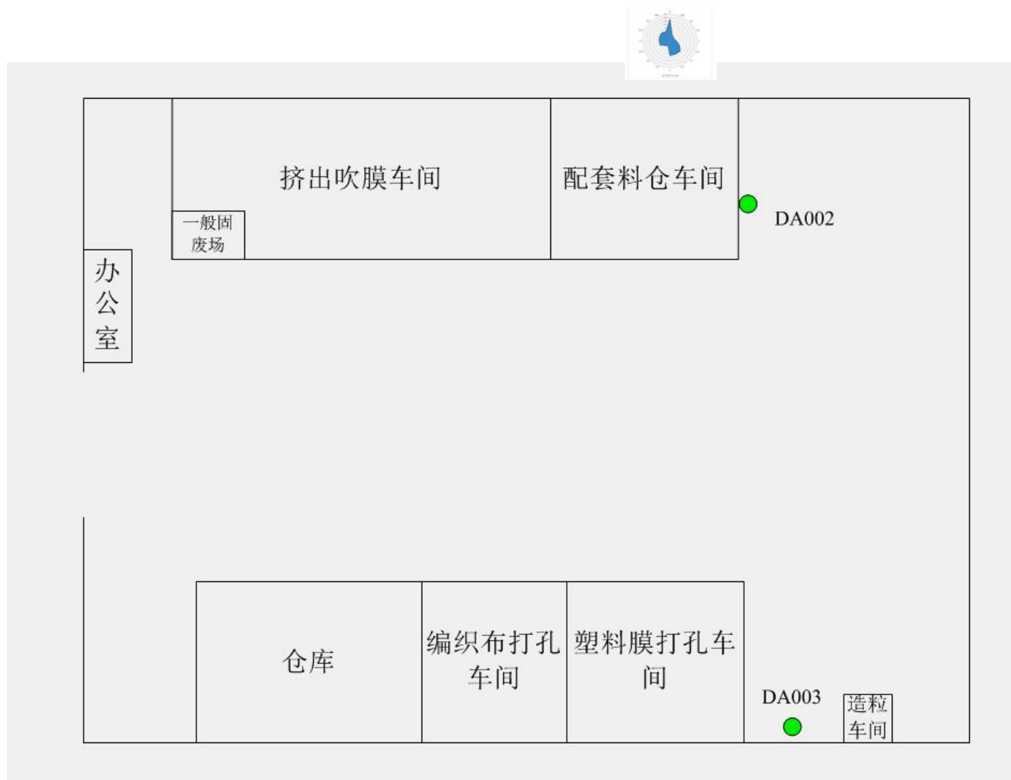
图3 项目厂区平面布置图
