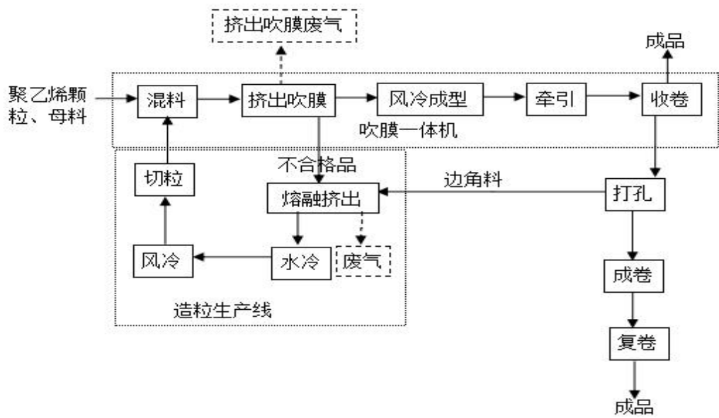
塑料薄膜生产工艺及产污环节图
